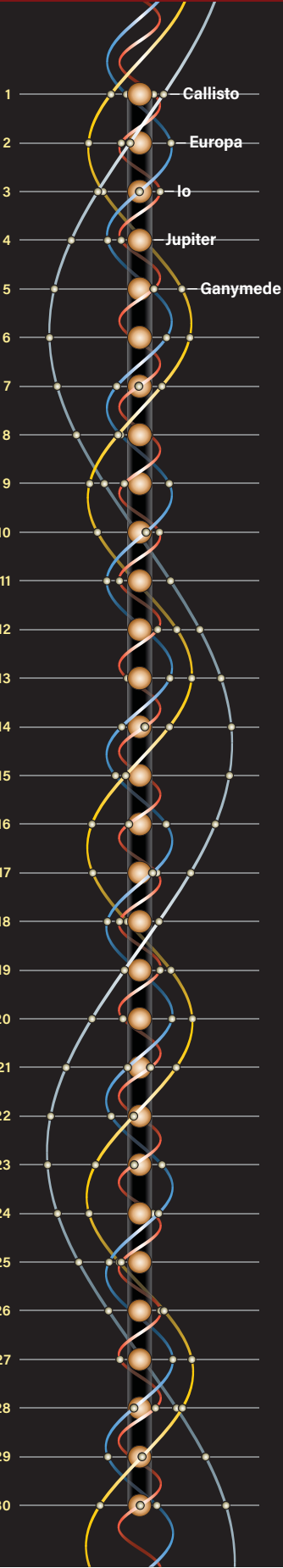
Ganymede
